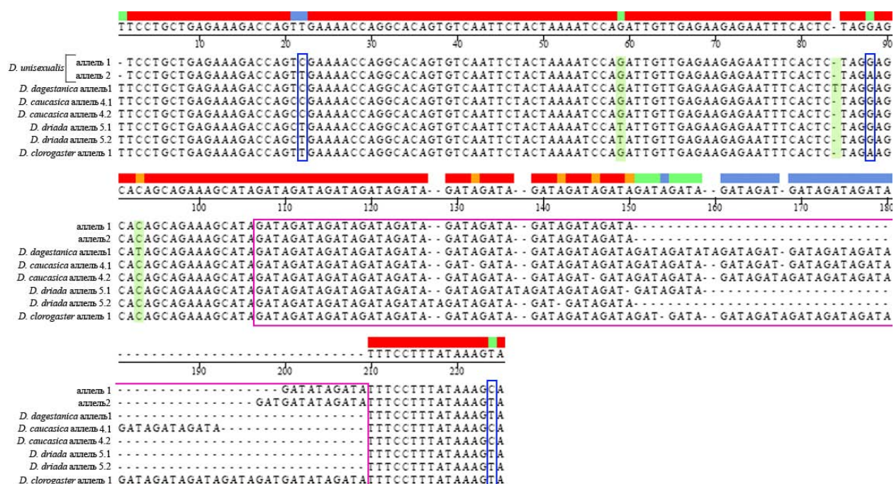
Рисунок 12. Нуклеотидные последовательности двух аллельных вариантов локуса Du281 D. unisexualis в сравнении с двуполовыми видами D. dagestanica , D. caucasica , D. driada , D. chlorogaster . Мутации во фланкирующих последовательностях ДНК выделены серым цветом. Однонуклеотидные замены, образующие гаплотипы, обведены прямоугольником. Микросателлитный кластер выделен рамкой.
